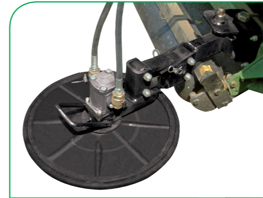
Kit disco con filo tagliaerba Central hydraulic mover Broyeur hydraulique central Fadenschneide
